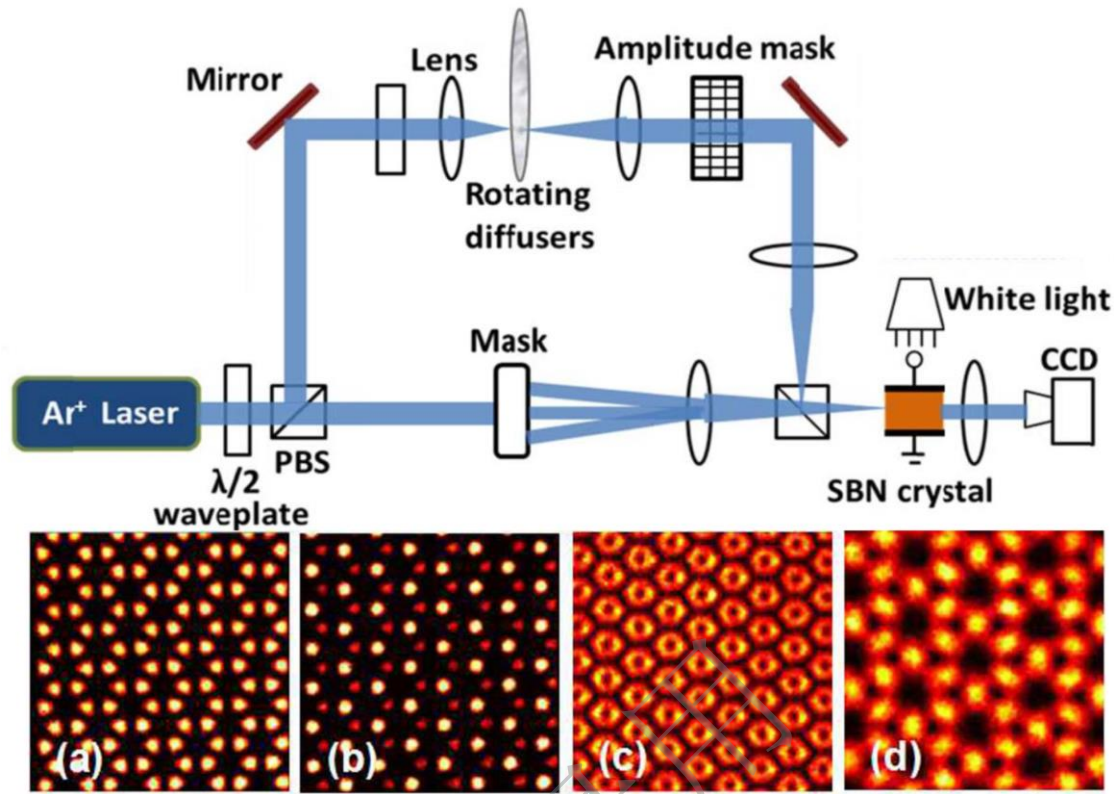
图 4 多光束干涉光诱导技术制备光子晶格 [80,83] 。第一排：实验光路图。PBS，偏振分光棱镜；Mask，掩模板；SBN，铌酸锶钡晶体。第二排：实验制作的典型光子晶格 (a) 蜂窝型光子晶格；(b) 对称破损的蜂窝型光子晶格；(c) 涡旋晶格；(d) Kagome晶格
