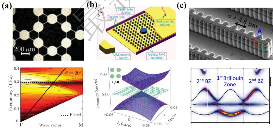
图 2 光子系统中平带研究的典型实例 (a) 上图为表面等离子激元平带的金属 Kagome 超构材料, 下图为对应的太赫兹波透射图, 存在一个全角度的无辐射平带 (水平虚线所示) [48] ; (b) 四方结构的全介质零折射率超构材料实现隐身效应实验装置, 下图为适当介质参数时得到的四方结构色散关系, 含有一个狄拉克锥与一个无色散平带 [50] ; (c) 一维“枕”型结构的微柱光学腔及其色散关系, 中间为平带 [51]
